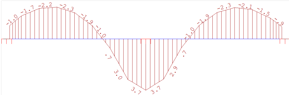
Fig 12. Momento na direção Y - Faixa do vão
