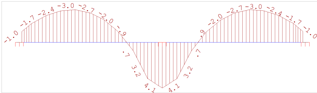
Fig 10. Momento na direção X - Faixa do vão
