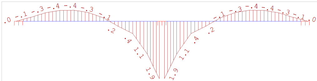
Fig 13. Momento na direção X - Faixa do apoio
