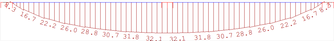
Fig 20. Momento na direção Y - Faixa do vão
