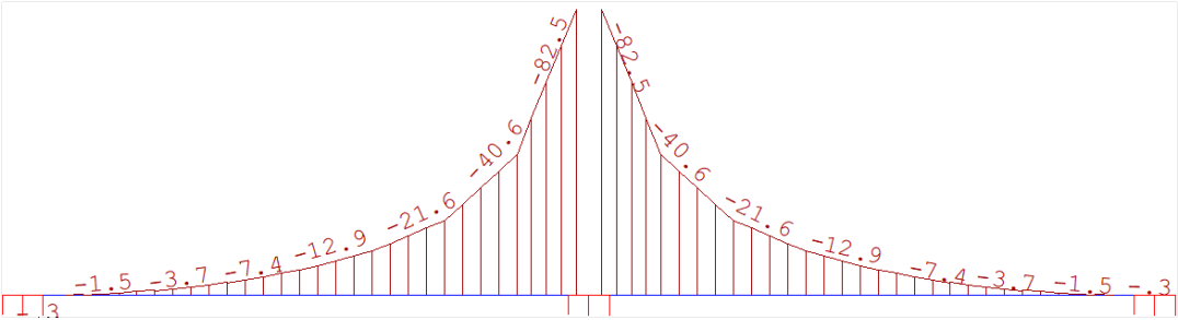
Fig 19. Momento na direção Y - Faixa do apoio
