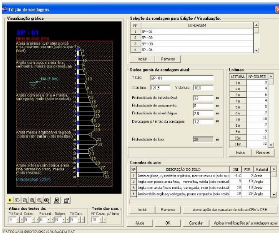
Figura 5 – Editor de sondagem do SISEs/TQS
